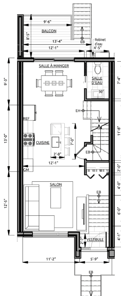
Étage 2 - 651 pi 2
